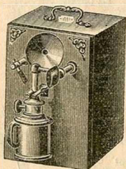
Allumoir portatif, à bouton, avec piles humides hermétiques. Prix..... 15.50
