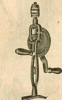
Porte-foret pour mèches de 0=001 à 0=013. 12.50
